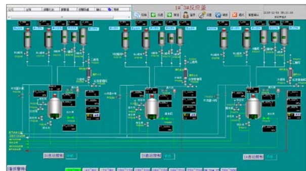
图9 反应釜组态画面
