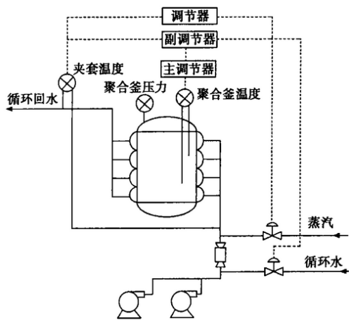
图4 聚合釜温度控制流程示意图
