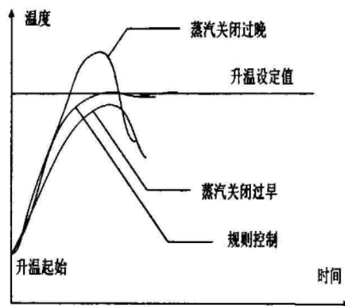
图5 升温控制效果
